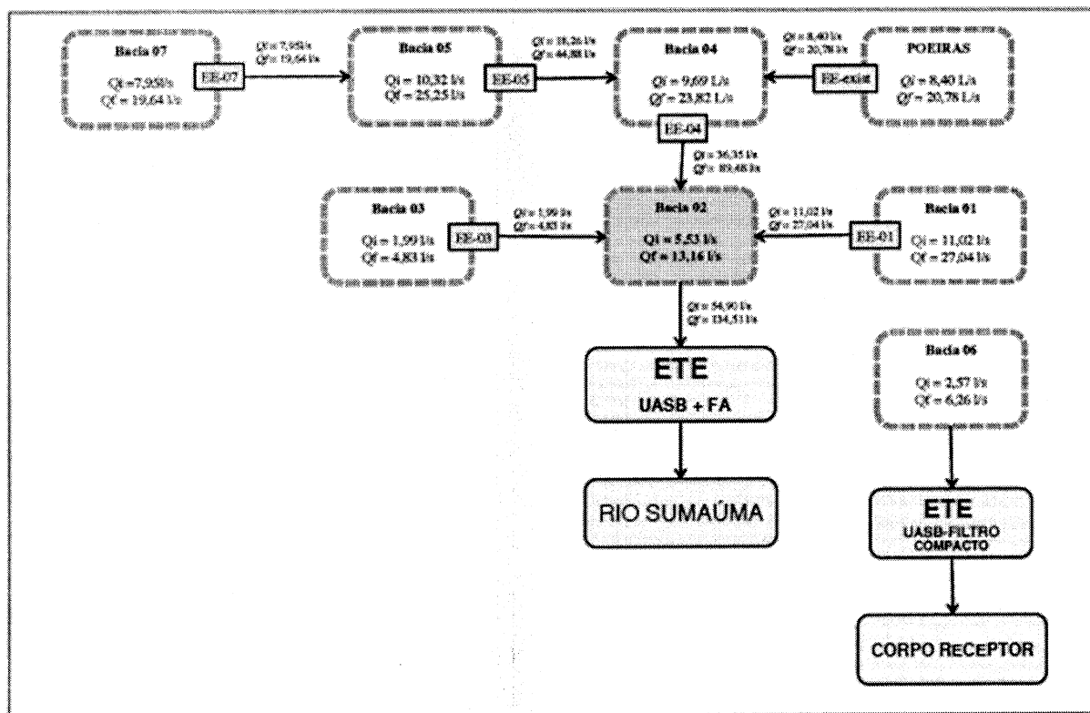
Figura 11: Fluxograma do Sistema de Esgotamento Sanitário em Implantação
